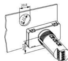
Рисунок 2 – Габаритные размеры корпуса ЩЗ
