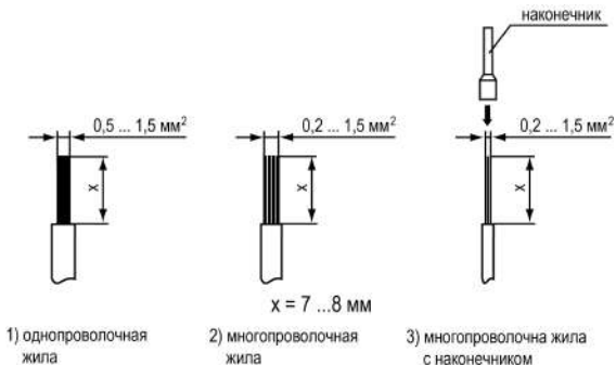
Рисунок 5 – Требования к сечениям жил кабелей и длине зачистки
